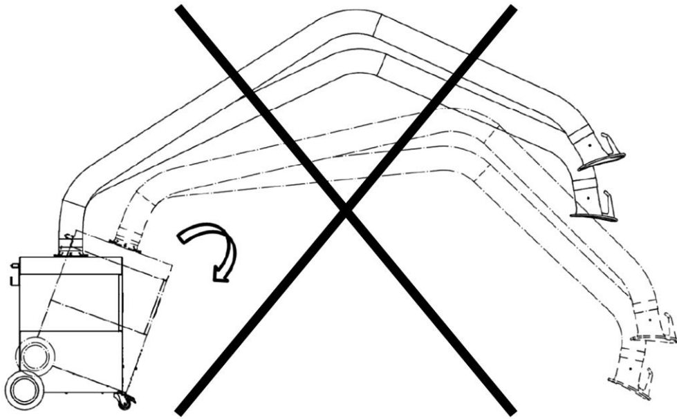
1. ábra: Az elszívókarok nem megfelelő pozicionálása
