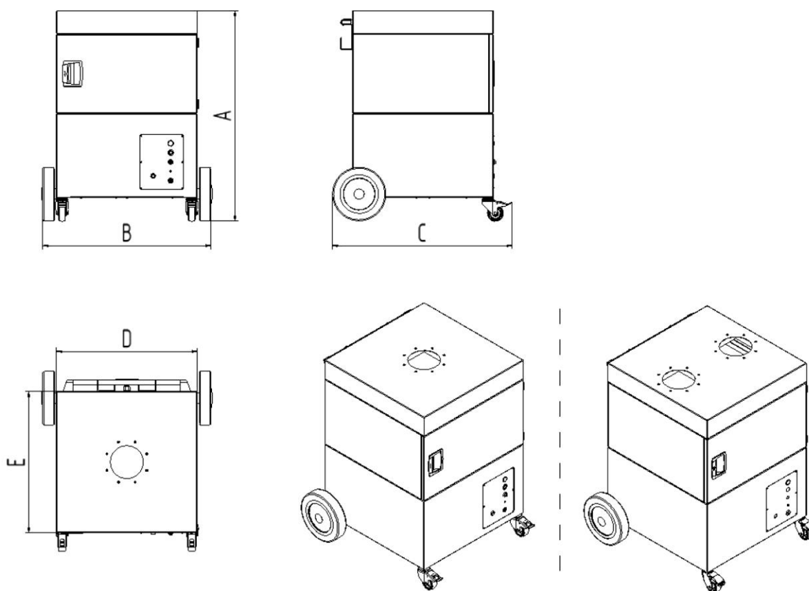
9. ábra: Mérettáblázat - 60650 + 60650DA
