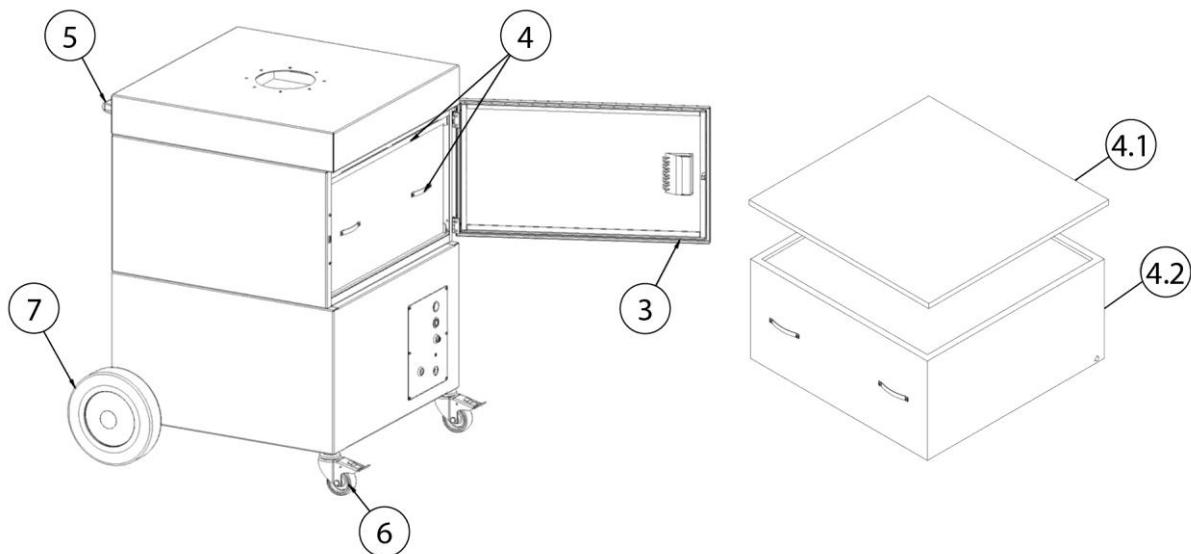
4. ábra: Összeszerelés
