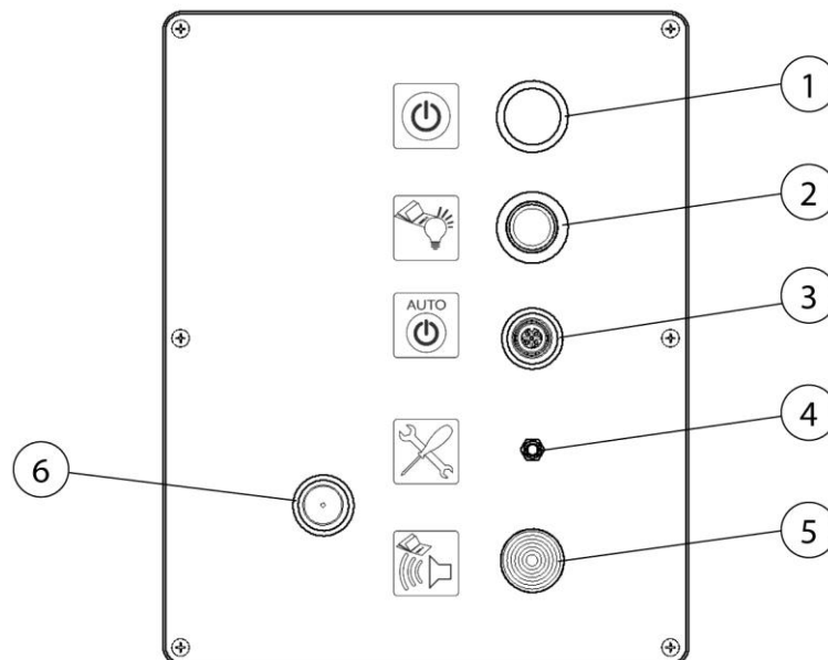
5. ábra: Kezelőelemek
